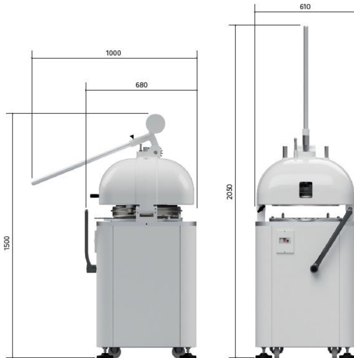
Główne wymiary półautomatycznej dzielarki – zaokrąglarki
